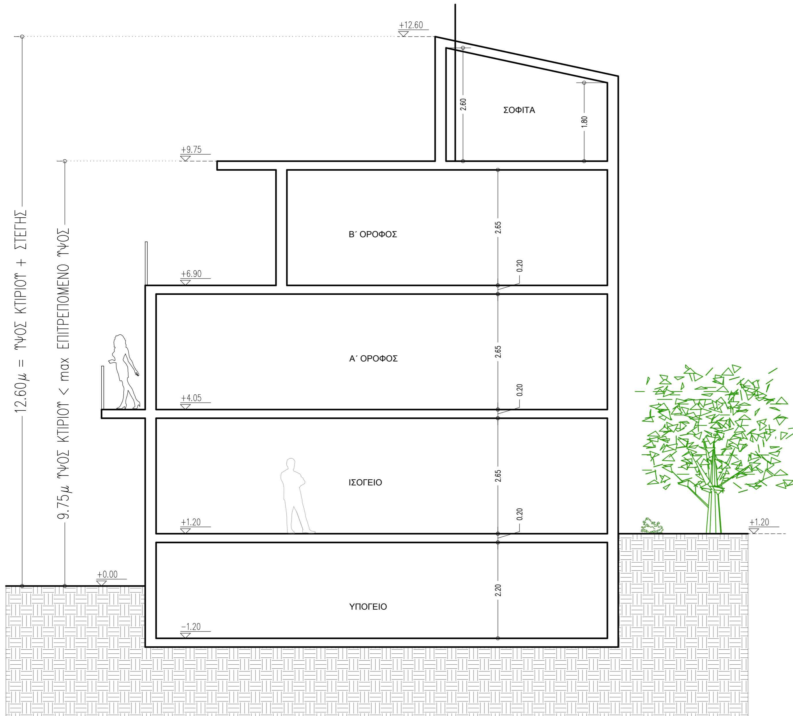
Τομή Β - Β' / Κλίμακα 1:50
