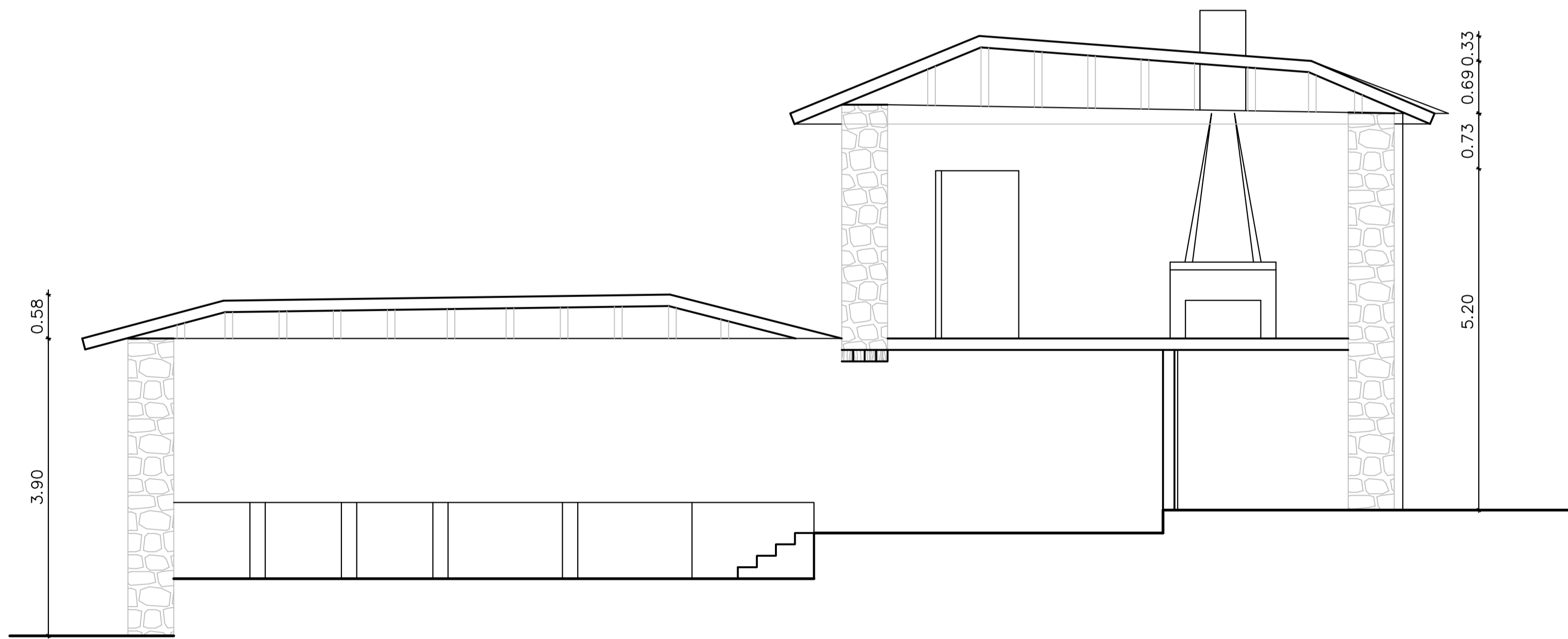
ΤΟΜΗ 3-3 ΒΥΡΣΟΔΕΨΙΟΥ
