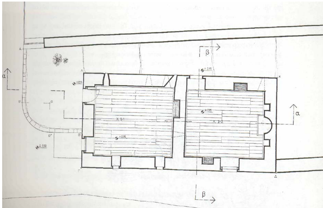
Σχεδιάγραμμα-δείγμα από τη μελέτη αποτύπωσης του κτηρίου του σχολείου (Αρχιτέκτονας Γεώργιος Γιαννίτσαρης, 1995).
